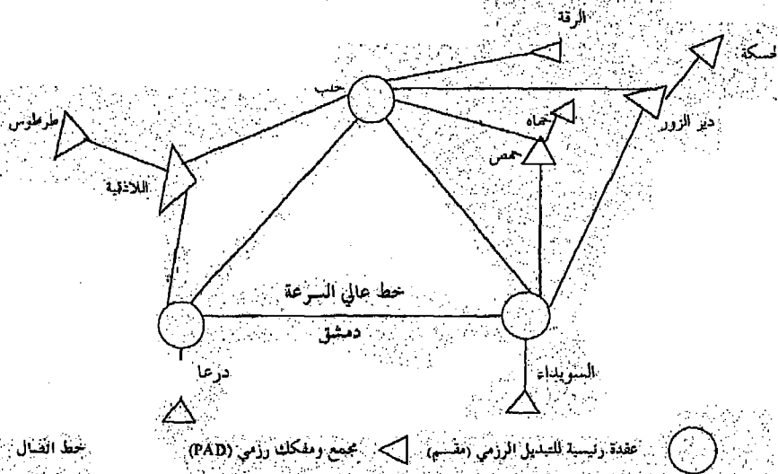
شكل 9-ب البنية العامة لشبكة Syriapac
